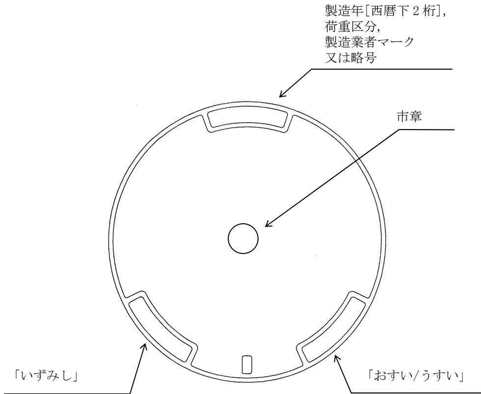
ふた表面図
