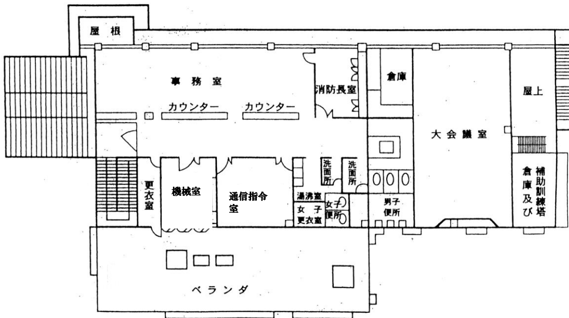
二階平面図 (560.00m 2 )
