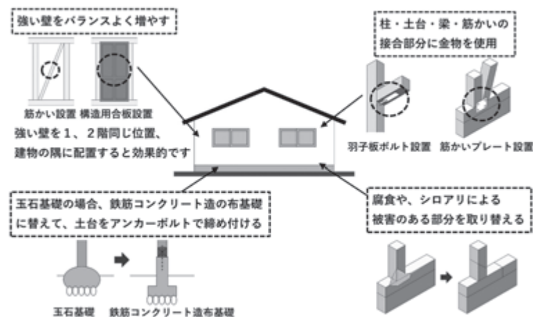
図：耐震改修工事の一例
