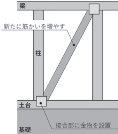
(耐震補強工事の例)
