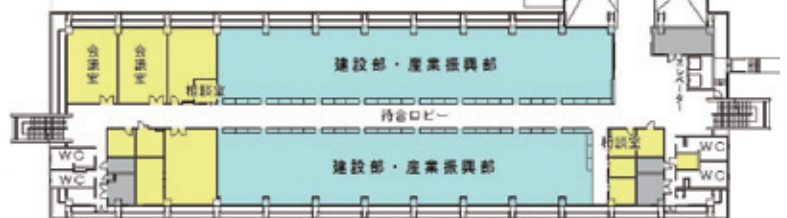
2階平面図
