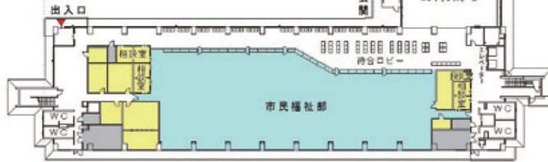
1階平面図
